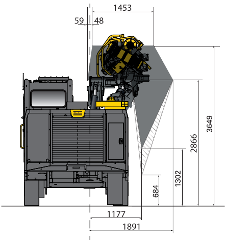
Khoan ngang thẳng mặt máy
