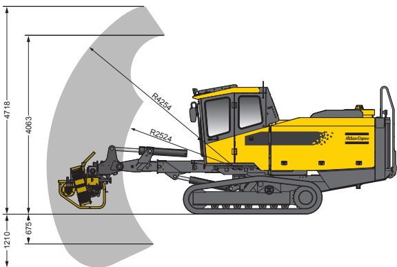
Khoan ngang sát đất (toe-hole)
